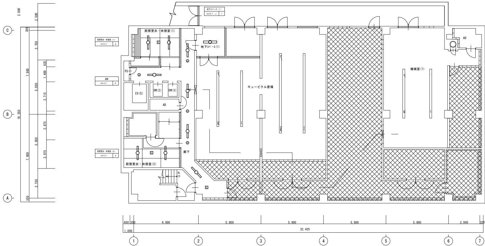
地階平面図 1 : 100
